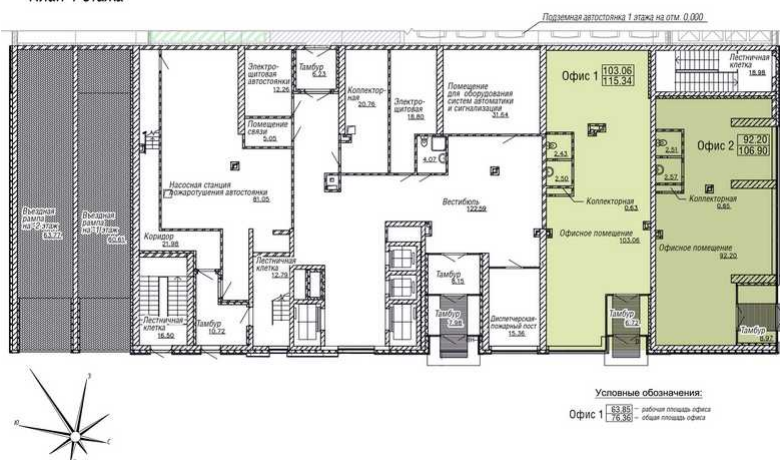
План 1 этажа
